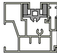
Doorsnede
