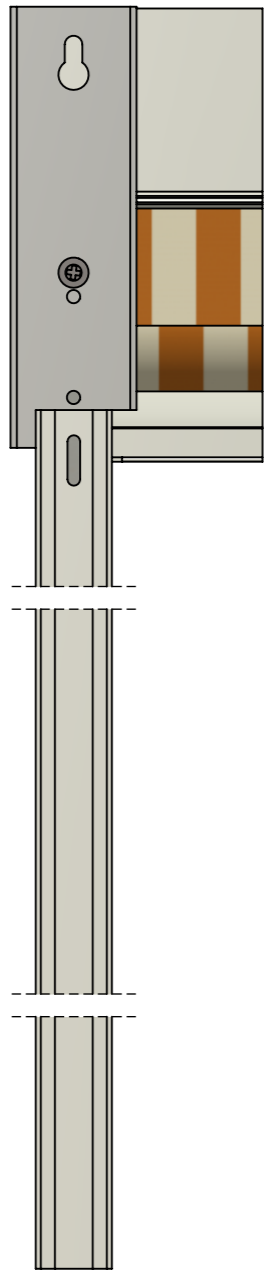
Achteraanzicht
